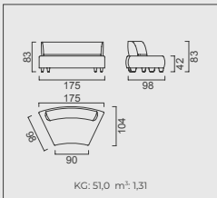
C Corner Module
