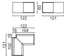
BUG 03 BETA CORNER TOP MODULE
