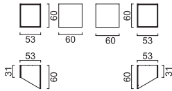
BUG 07 BETA ANGLED TOP MODULE
